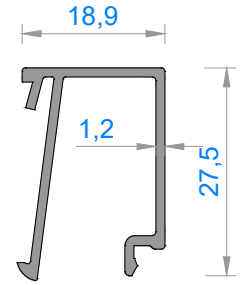
Sistem Kodu 9119* Ağırlık (kg/mt) 0,275
