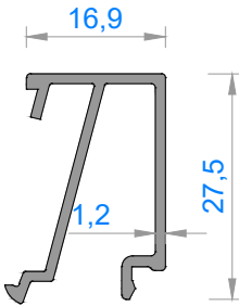
Sistem Kodu 9110* Ağırlık (kg/mt) 0,277
