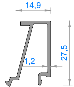
Sistem Kodu 9112* Ağırlık (kg/mt) 0,255
