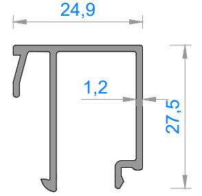
Sistem Kodu 9010 Ağırlık (kg/mt) 0,309
